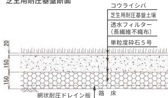
芝生用耐圧基盤断面
